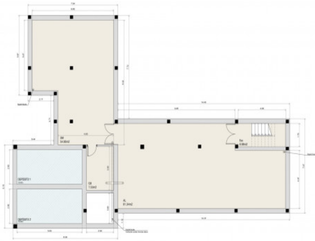
SUPERFICIE CONSTRUIDA DE GOTANCO=710M2 PLANTA GOTANCO E: 1/50
